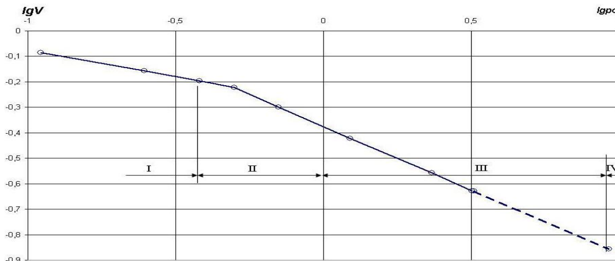
Рисунок 1 - Зависимость относительного объема пара от давления сжатия
