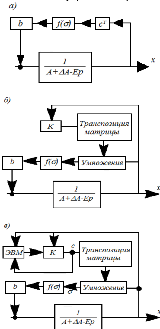
а) исходная система; б) самонастраивающаяся система; в) самообучающаяся система.
