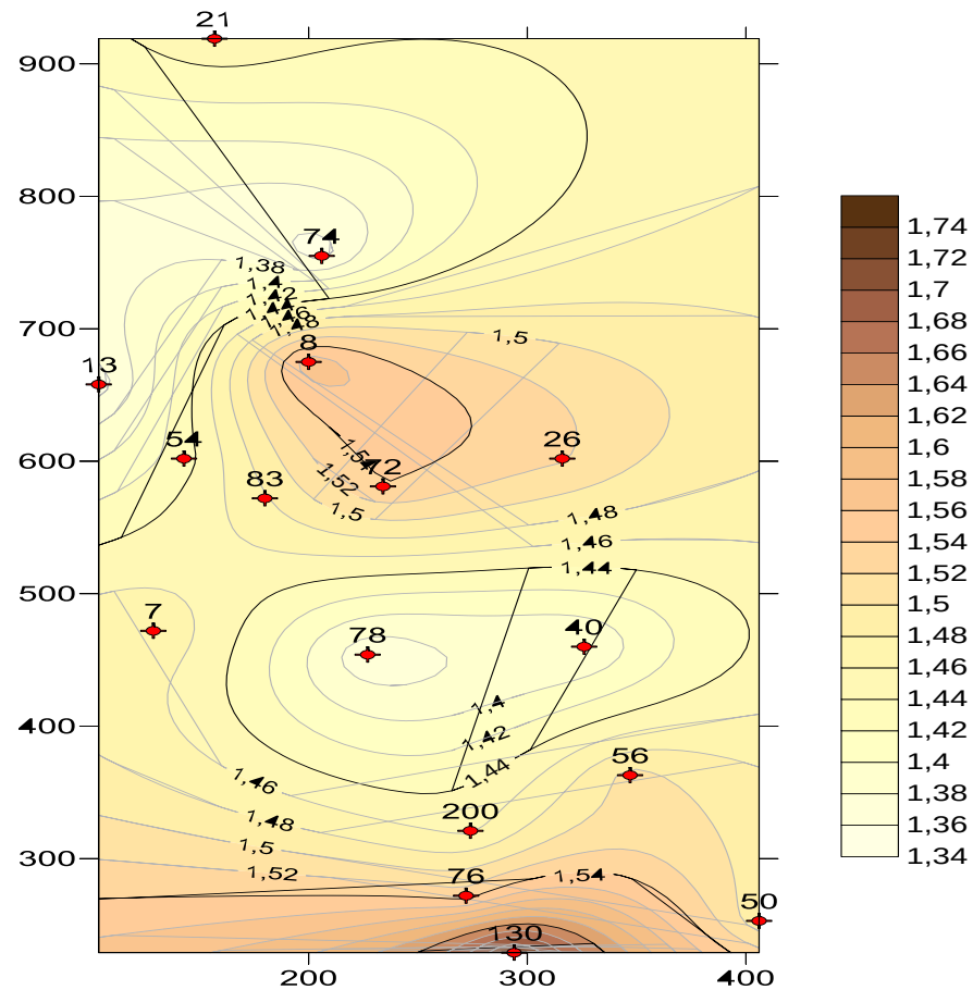
Рис. 2. Распределение плотности бурового раствора на месторождении Бахар (Сураханская и Сабунчинская свиты)
